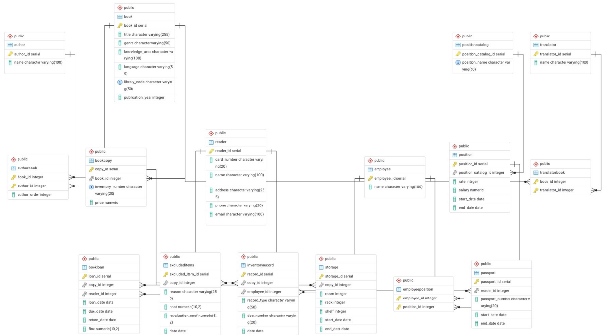
Рисунок 1 Схема логической модели базы данных
